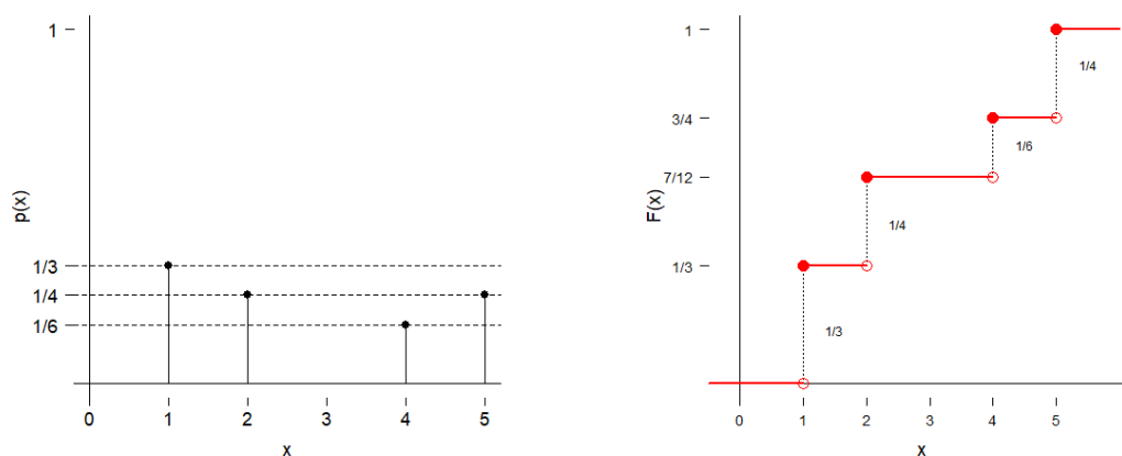
Obr. 1: Pravděpodobnostní a distribuční funkce k příkladu 3.6
